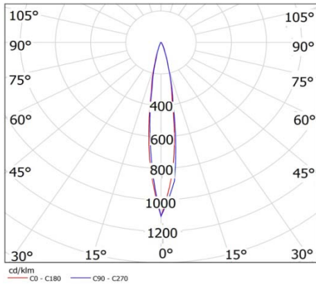
25°配光曲线图
