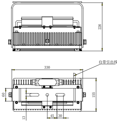
LF21XX 安装尺寸图 (单位: mm)
