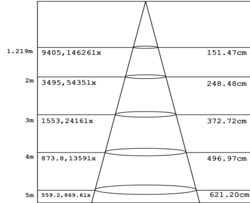
15°照度锥形图
