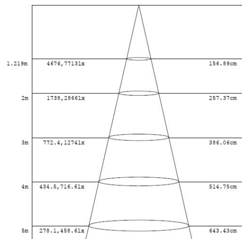
60°照度锥形图
