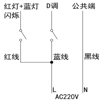
图一 声光分开报警
